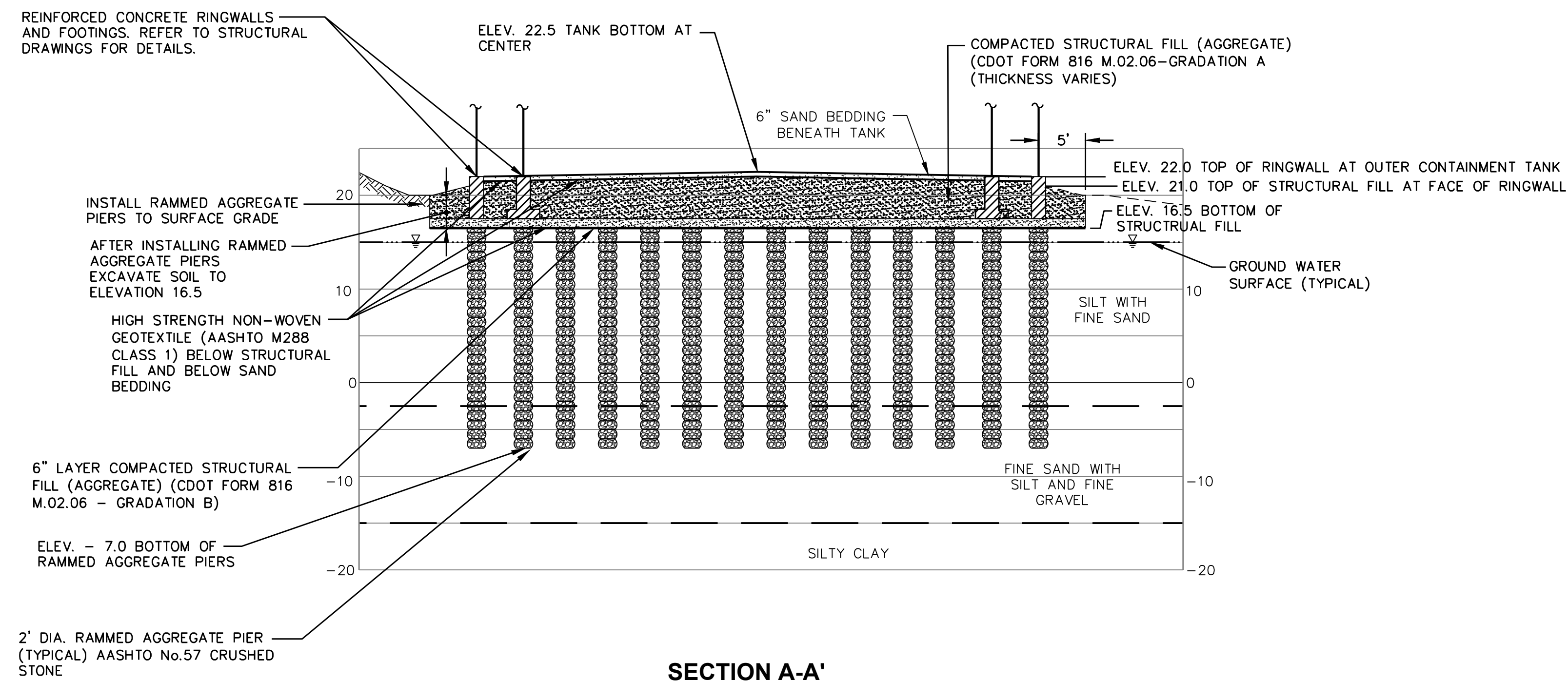
SECTION A-A'
